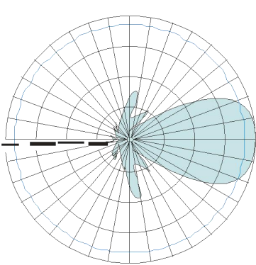
H-Plane
