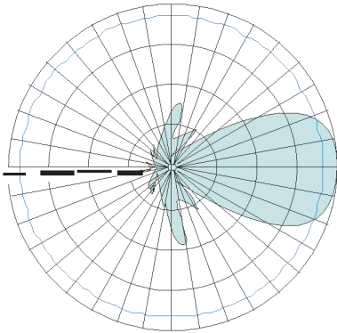
E-Plane
